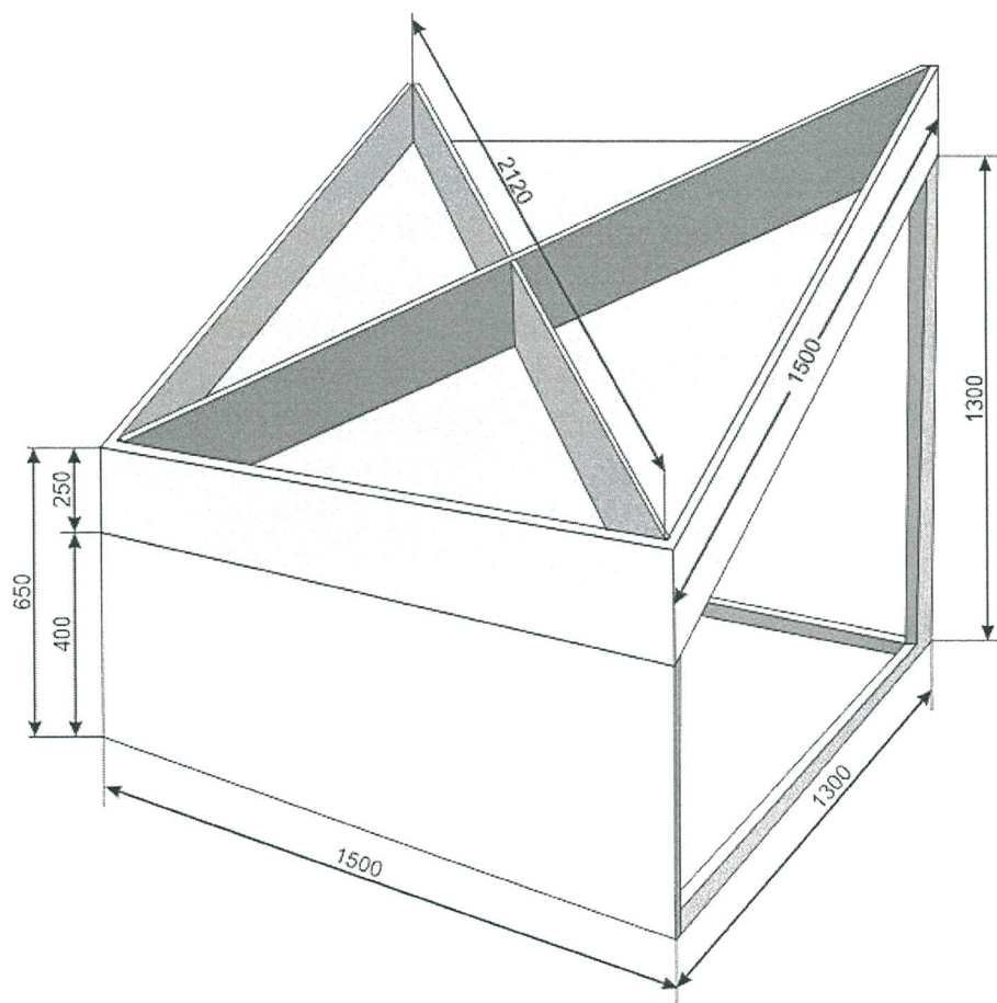
Рис.1. Внешний вид стеллажа для выкладки товара
